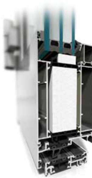
Tür MB-86 Aero
